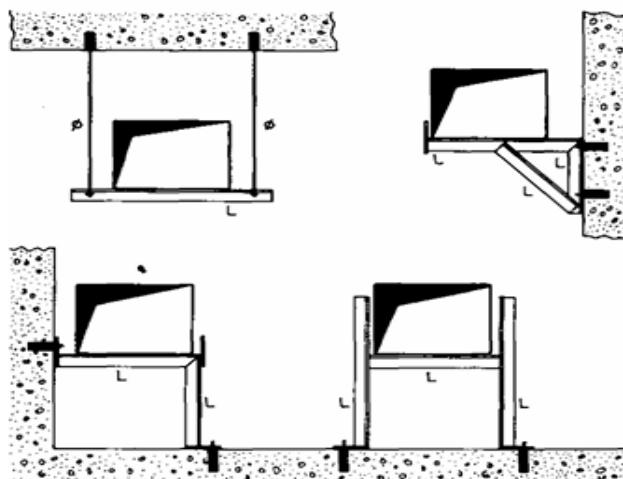
Σχήμα 7 - Στήριξεις/αναρτήσεις αεραγωγών
