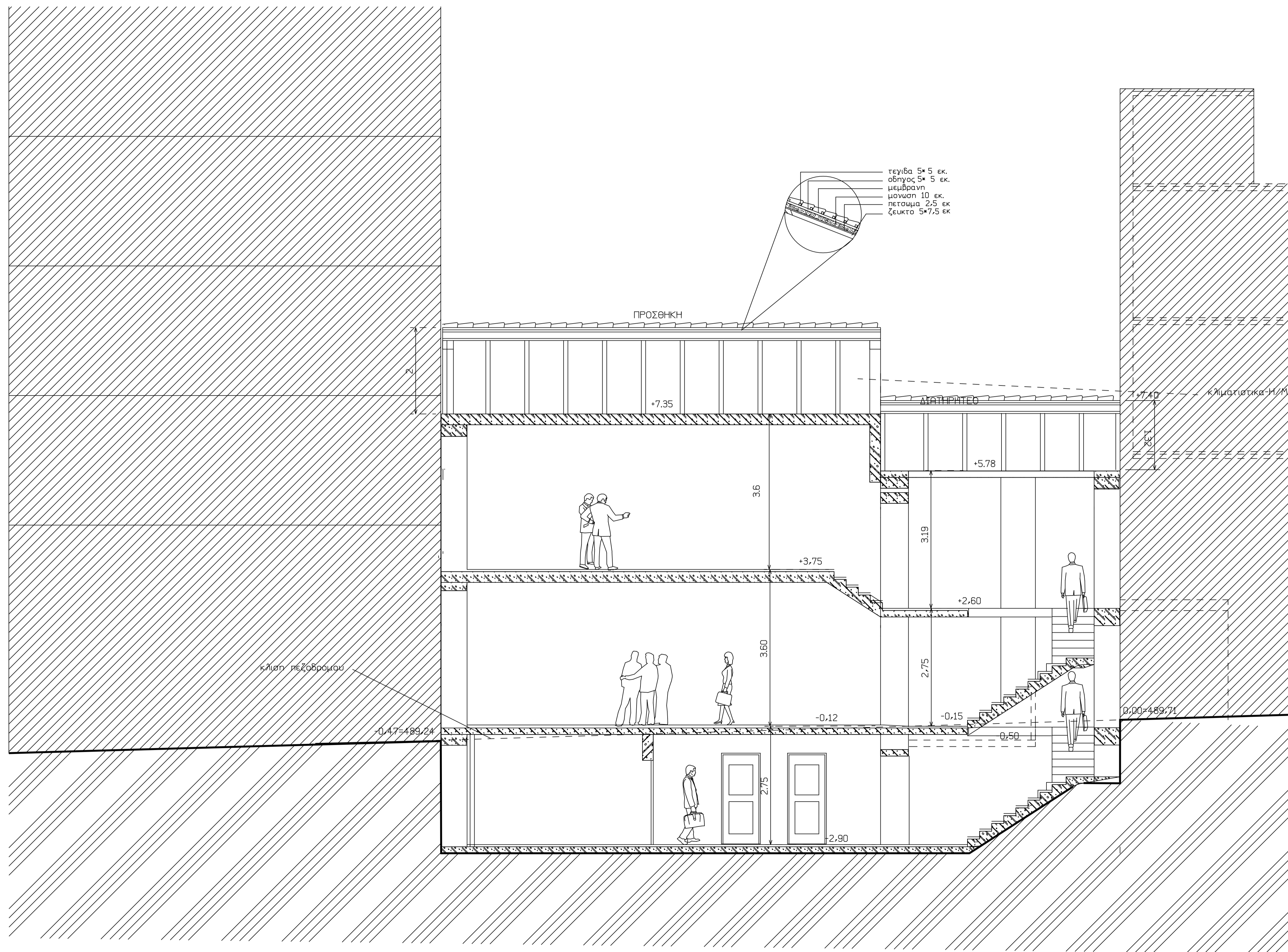
τομή α-α 1/50
